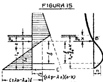
FIGURA 15 Estudio de un estacado anclado suponiendo encastramiento inferior por medio de la viga de reemplazo, determinación de la ficha.
