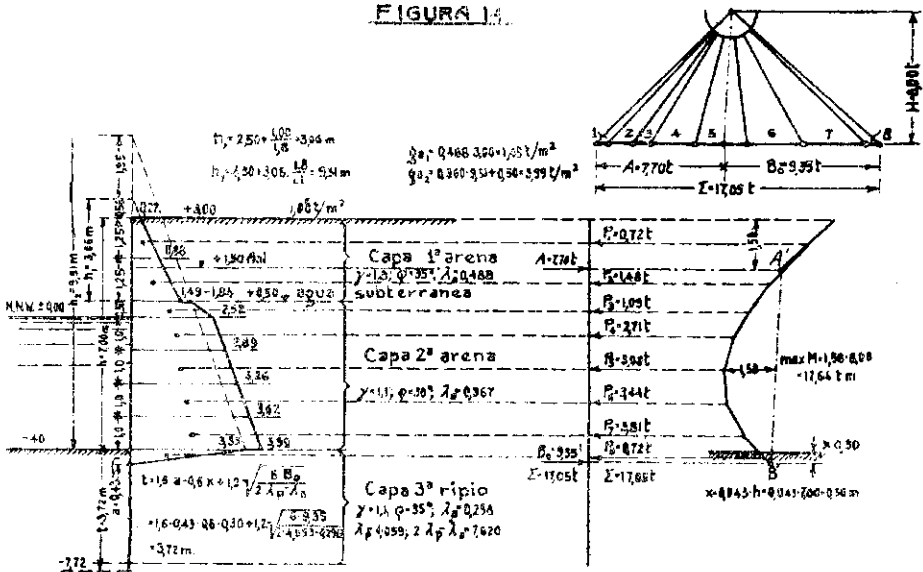
Estudio de un estacado anclado, suponiendo encastramiento inferior por medio de la viga de reemplazo.
