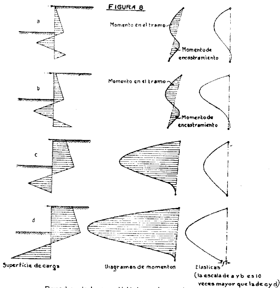
Pared anclada con distintas sobrecargas
